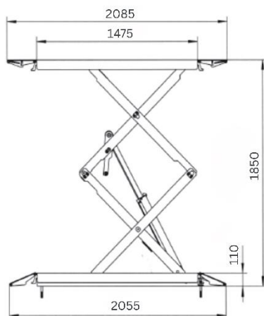
Podwójne siłowniki
